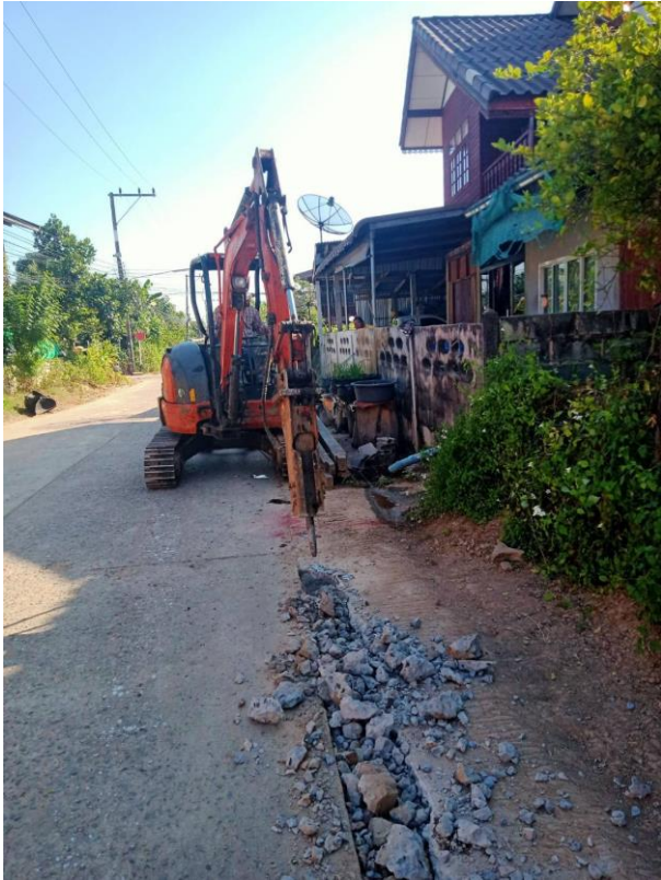
โครงการก่อสร้างขยายเขตวางท่อประปาเริ่มจากบ้านนายสหทรัพย์ ภูแอบหิน ถึงบ้านนายหนูคล้าย รุ่งริ่ง หมู่ที่ ๑ อำเภอห้วยเม็ก จังหวัดกาฬสินธุ์
